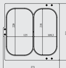
قالبی ستاندارد Standard Mold
