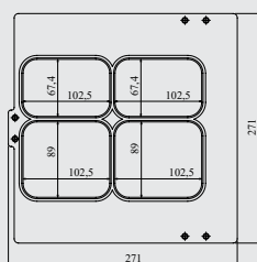
قالبی تورکی Turkish Mold
