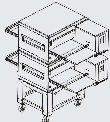
سیستمی سه‌ریه‌خۆ بۆ هه‌ردوو قات Two Floor Modular System
